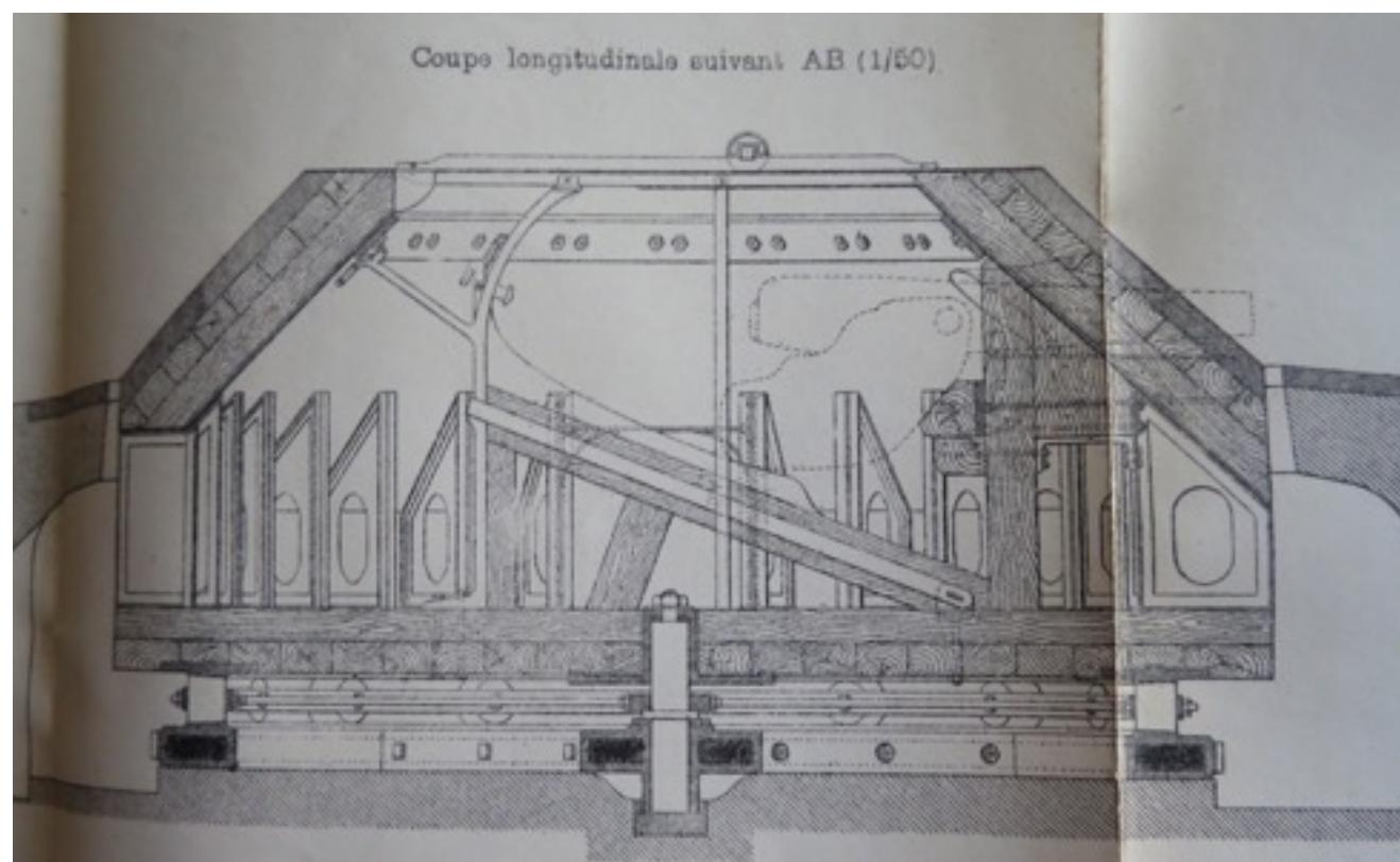
Afb. 28: Doorsnedes van een koepel die mogelijk voor bastion Oranje gepland was, zoals afgebeeld in "Etude des Tourelles Cuirassees Tournantes" door Mougins uit 1873. Dit type koepel is ook toegepast op de forten in Antwerpen (privécollectie auteur)
