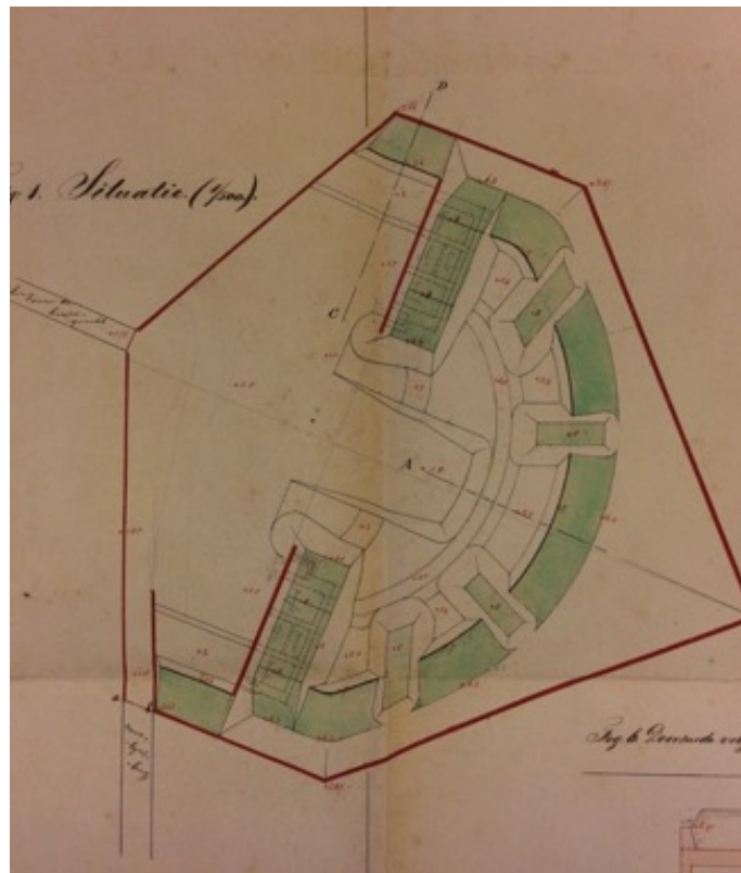
Afb. 29: De plattegrond van ravelijn 6 van 28 april 1873. Er is slechts sprake van twee kleine kazernes annex remisegebouwen en geschutsopstellingen in de openlucht. De kazematten zijn geheel uit het plan verdwenen (NA 2.13.01-3608-71G)
