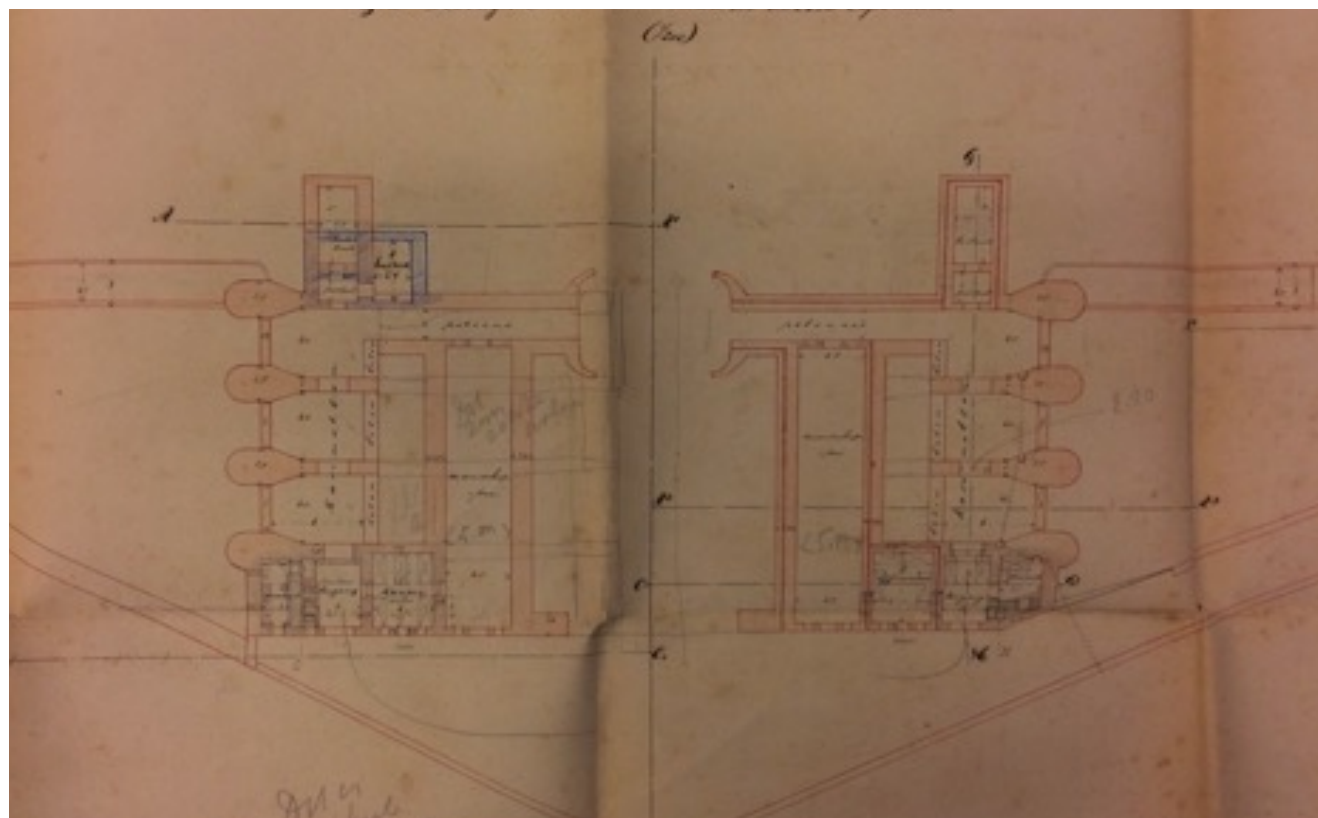
Afb. 6: Detail van de kazemattengebouwen (NA.2.13.01-3582-53G). Achter de kazematten liggen manschappenverblijven. Er tussen ligt een ruimte die gevuld werd met aarde. Als commentaar staat op de tekening "dit zijn echte hollen" geschreven bij de manschappenverblijven. Ze hadden ook slechts een smalle gevel waar daglichtopeningen gemaakt konden worden.
