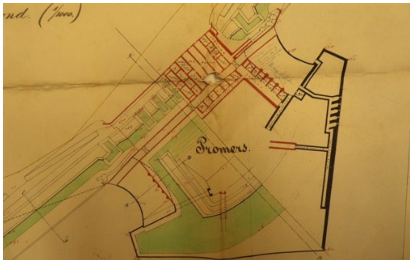
Afb. 13: Detail van het bastion Promers. In de keel van het bastion komt een grote kazerne te liggen. Dwars door de kazerne loopt een gracht die aansluit op de vestinggracht. De kazernes aan weerszijden van deze gracht zijn bereikbaar via rolbruggen. In de flanken van het bastion zijn kazemattengebouwen aangebracht (NA 2.13.01-3583-56G)
