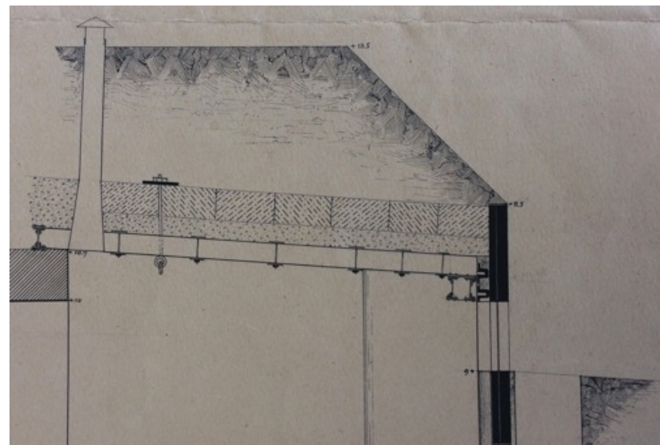
Afb. 27: Detail van de doorsnede van de geschutstanden (NHA 548, inv. nr. 192)
